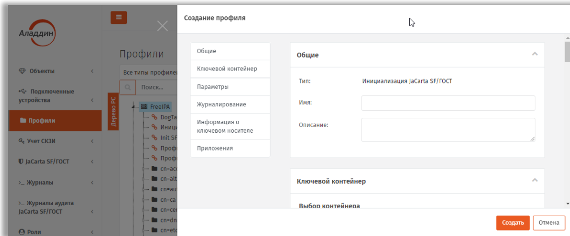
Рис. 90 – Вкладка Общие
