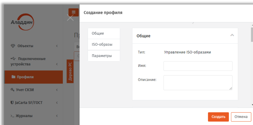
Рис. 100 – Вкладка Общие
