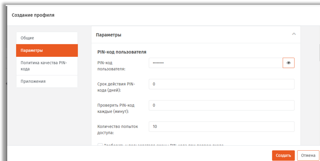
Рис. 87 – Вкладка Параметры
