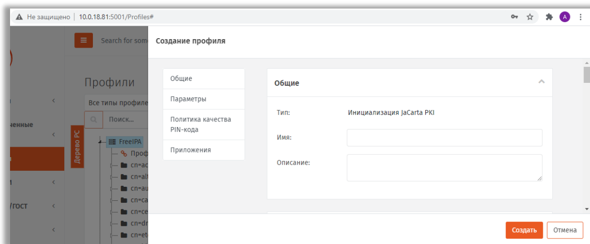
Рис. 86 – Вкладка Общие
