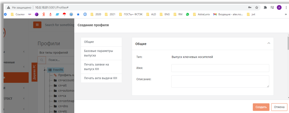
Рис. 83 – Вкладка Общие
