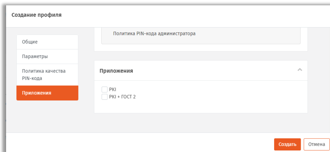
Рис. 89 – Вкладка Приложения
