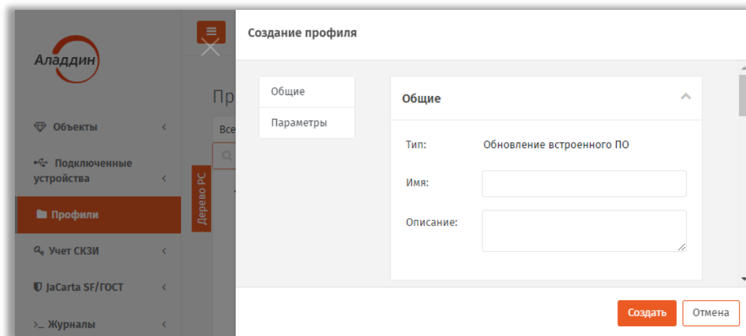
Рис. 102 – Вкладка Общие
