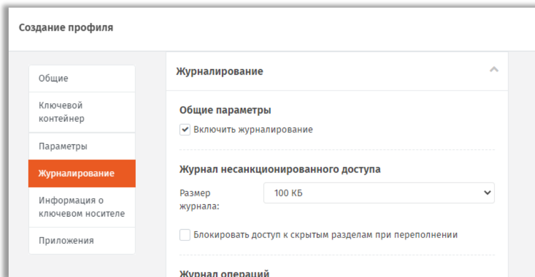
Рис. 93 – Вкладка Журналирование
