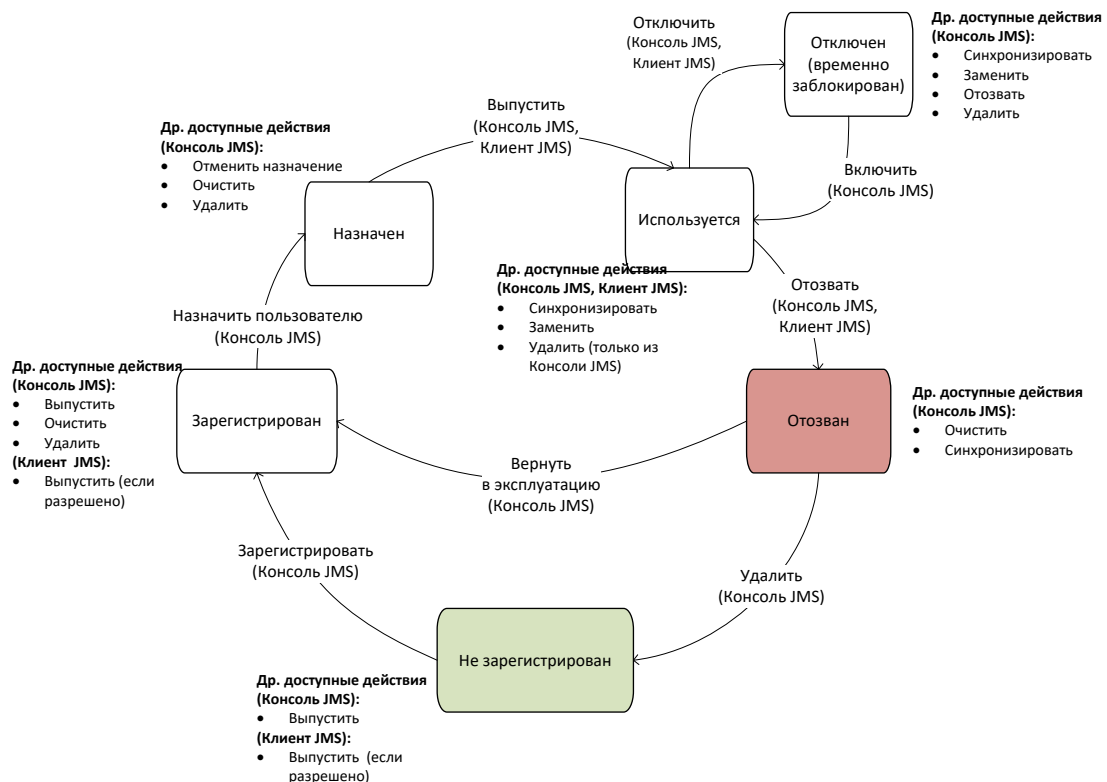
Рис. 21 – Диаграмма жизненного цикла ключевого носителя (электронного ключа/ЗНИ)
