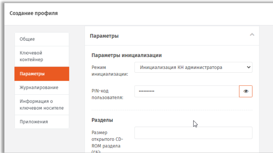
Рис. 92 – Вкладка Параметры
