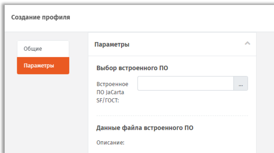
Рис. 103 – Вкладка Параметры
