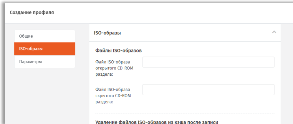
Рис. 101 – Вкладка ISO-образы
