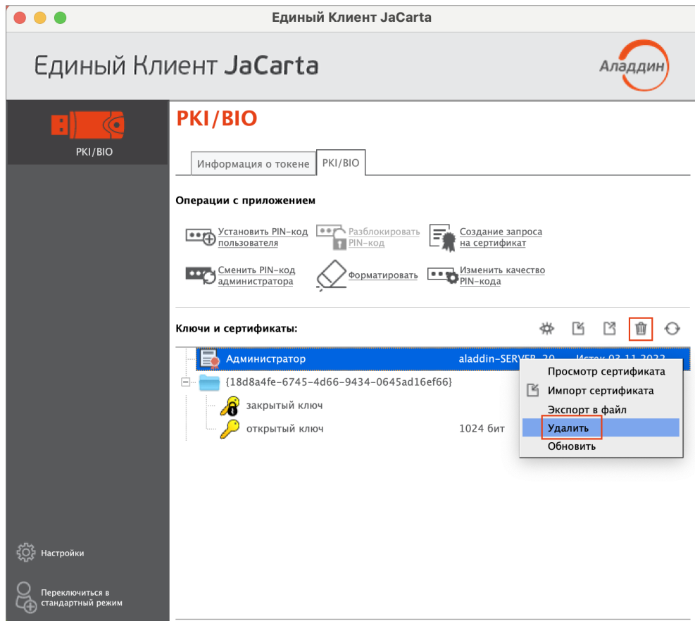
Рисунок 50 - Единый Клиент JaCarta. Кнопки перехода к удалению данных
