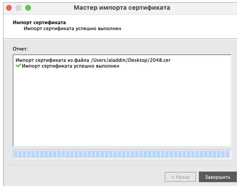
Рисунок 45 - Мастер импорта сертификата. Сообщение об успешном импорте сертификата
